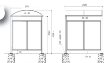
Schemat konstrukcji.
